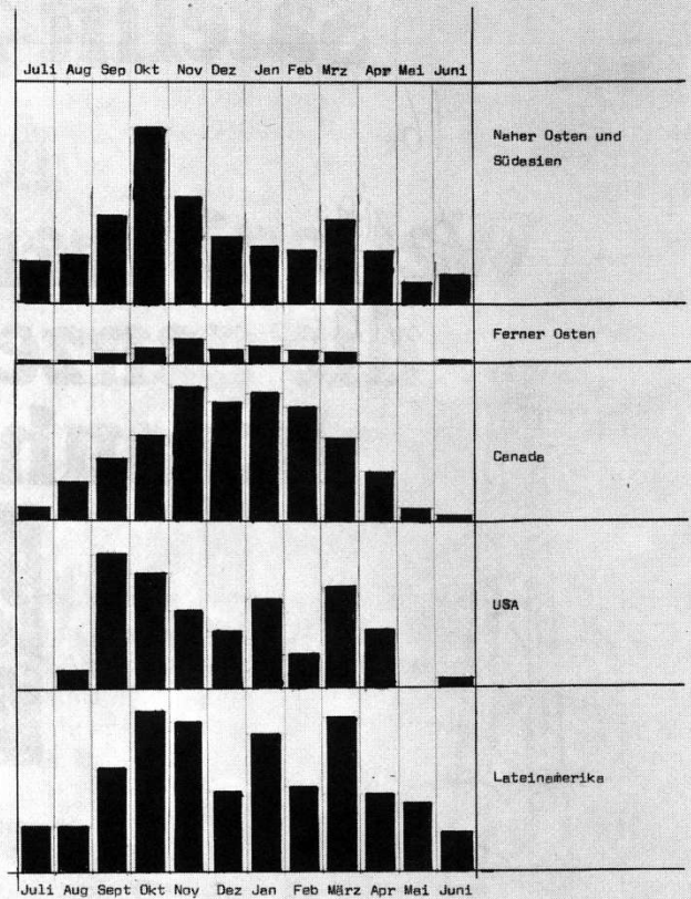
Abb. 2: Jahresgang der Empfangsmöglichkeiten von Mittelwellensendern aus Übersee (auf der Grundlage in Deutschland geloggtter Stationen)
