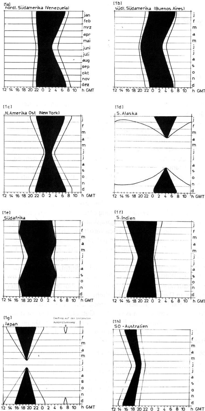
Abbildung 1: Jahreszeitlicher Gang der Zeitspanne mit Marlichkeit fur Mittelwellenfernempfang fur acht ausgewahlte Senderstandorte. Empfangerstandort: Suddeutschland. (Einzelheiten siehe Text)
